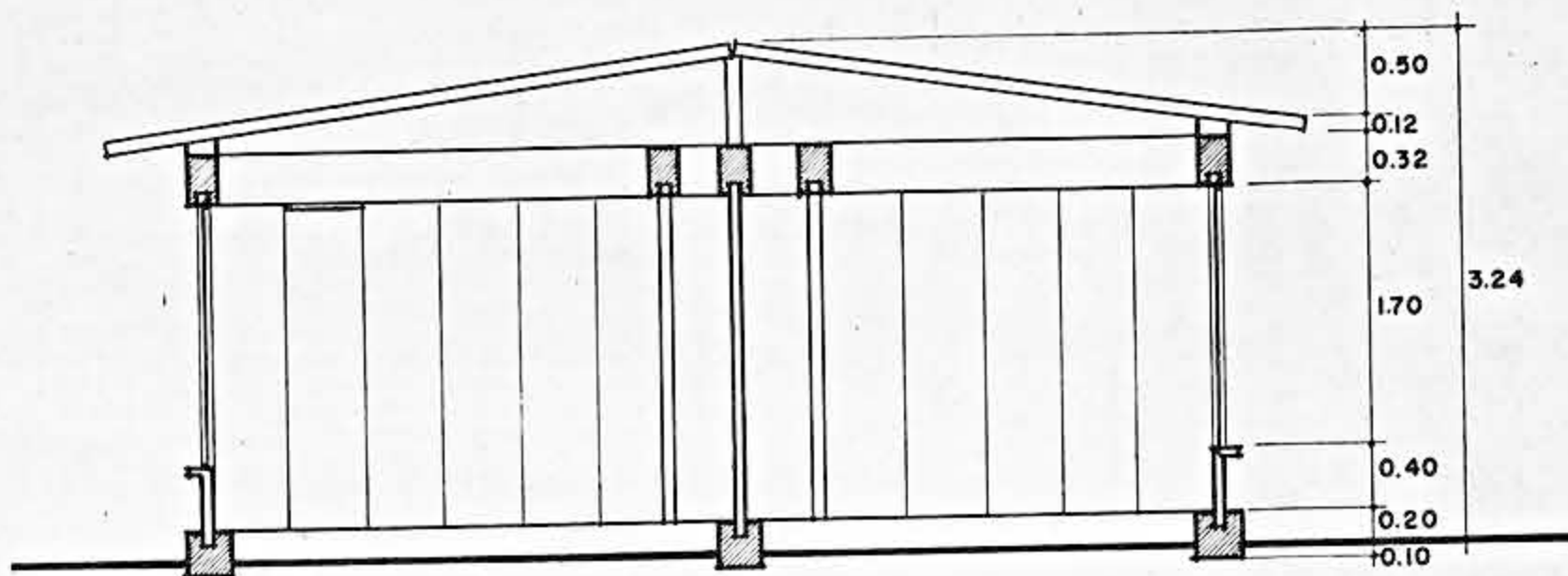
CORTE ESQUEMATICO
