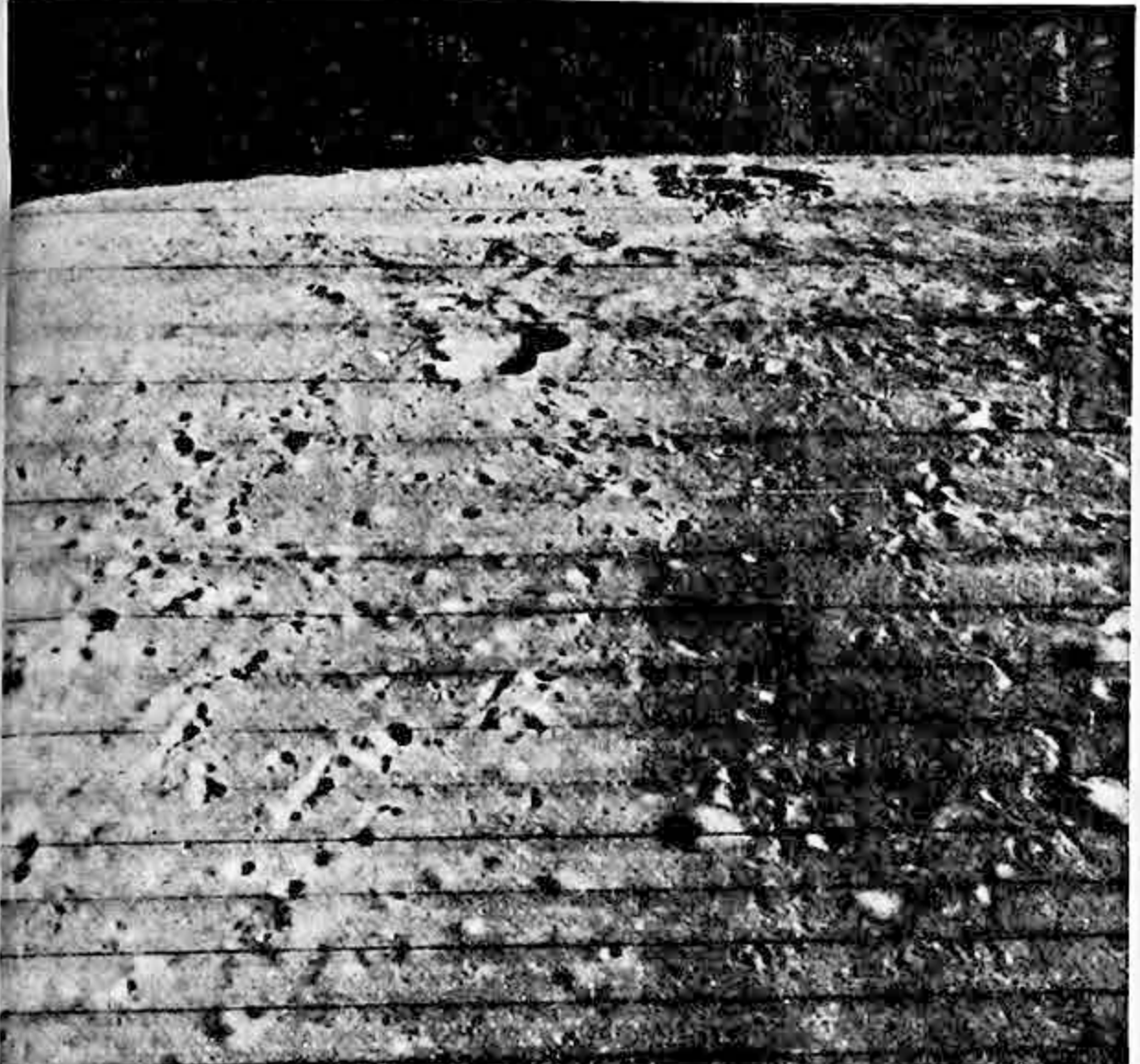
Una vista oblicua de la Luna. Fue captado por las cámaras del Orbiter Lunar II. El cráter Copérnico está próximo al horizonte. El Orbiter Lunar se encontraba a 28.4 millas sobre la superficie del satélite cuando fue captada la presente fotografía (AP Wirephoto)
