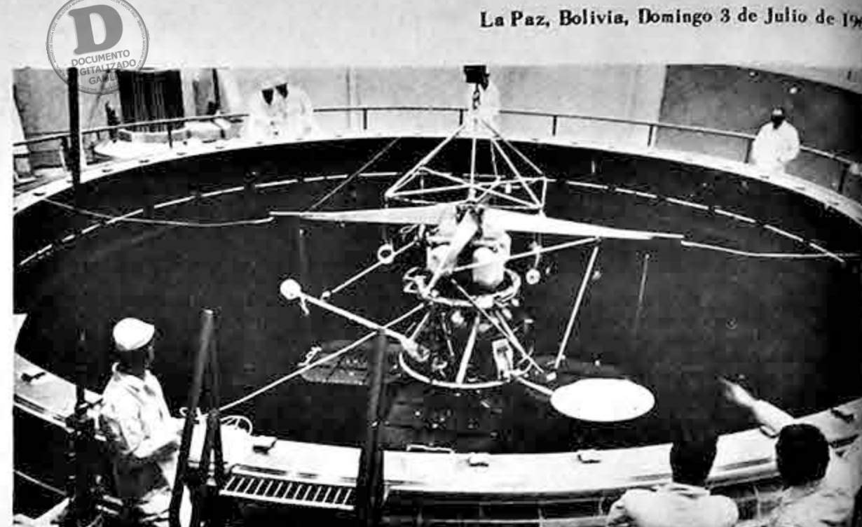
ORBITADOR LUNAR.- La nave espacial orbitador lunar con las antenas y paneles solares abiertos es colocado en una cámara de prueba que simula los cambios extremos de temperatura y las condiciones cercanas al vacío absoluto en la superficie lunar. El orbitador lunar ha sido diseñado para fotografiar posibles sitios de descenso de los futuros vuelos tripulados norteamericanos del Proyecto Apolo.
