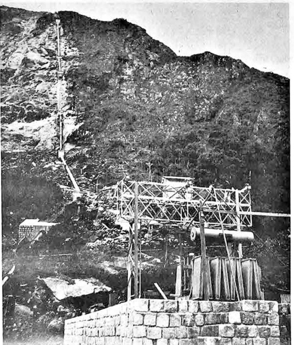
La subestación eléctrica de Chururaqui, con el transformador de 14.500 KVA y 66 KV y la estructura metálica de operaciones y la cañería de presión.
