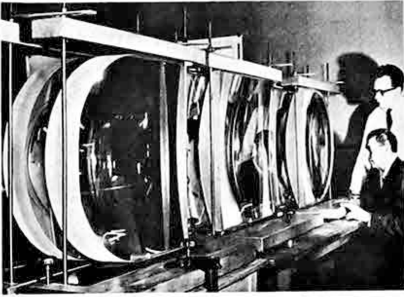
Stuttgart.- Tres lentes dobles de enormes dimensiones, producidas en la fábrica más grande de artículos ópticos de Alemania Occidental, probaron su eficacia en el Centro Europeo de Investigación Nuclear en Ginebra. Cada una de las lentes condensadoras de 70 cm. de diámetro y 160 kilos de peso tiene el objeto de conducir en una cámara de burbujas de hidrogeno, una luz, emanada por tres lámparas de centelleo de alta potencia, concentradamente a través de la cámara de burbujas a unos aparatos fotográficos. El hidrogeno líquido que se encuentra en la cámara, cerrada herméticamente, se halla bajo una presión de 6 at., mediante una disminución de corta duración de la presión, el hidrogeno licuefacto adquiere un estado "sobrecalentado". En este momento es pasada una corriente de partículas elementales las que producen caminos de burbujas que pueden ser fotografiados por los físicos nucleares. De la evaluación de tales experimentos se sacan valiosos conocimientos para la física nuclear. Nuestra foto muestra las tres lentes dobles durante el control en la fábrica alemana poco antes de ser expedidas a Ginebra.
