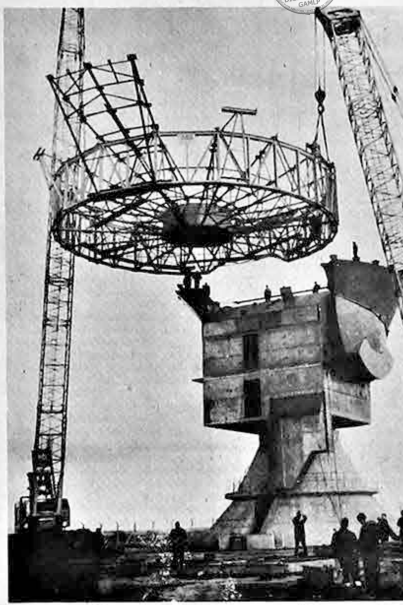
Estructura de acero con un peso de 35 toneladas que servirá para instalar un radio telescopio de 30 metros de diámetro en Chilbolton, New Hampshire. El radio telescopio servirá para investigar todos los problemas que se relacionan con los satélites (AP Wirephoto)
